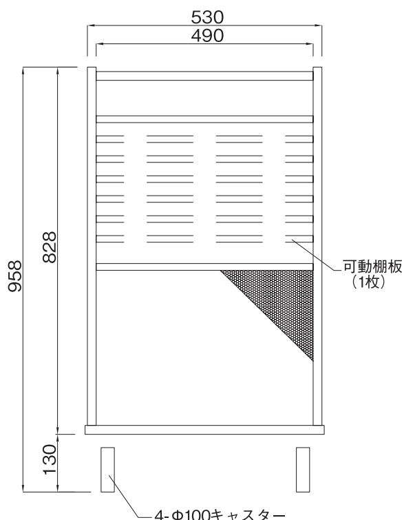
【正面図】
