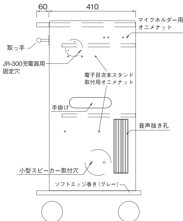
【側面図】
