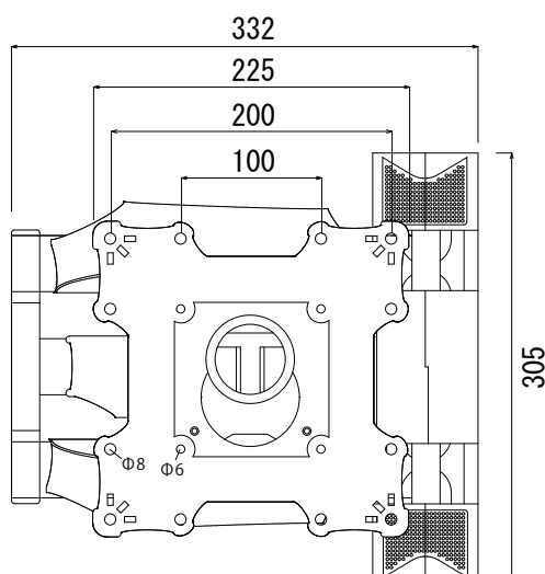
【ディスプレイ側】
