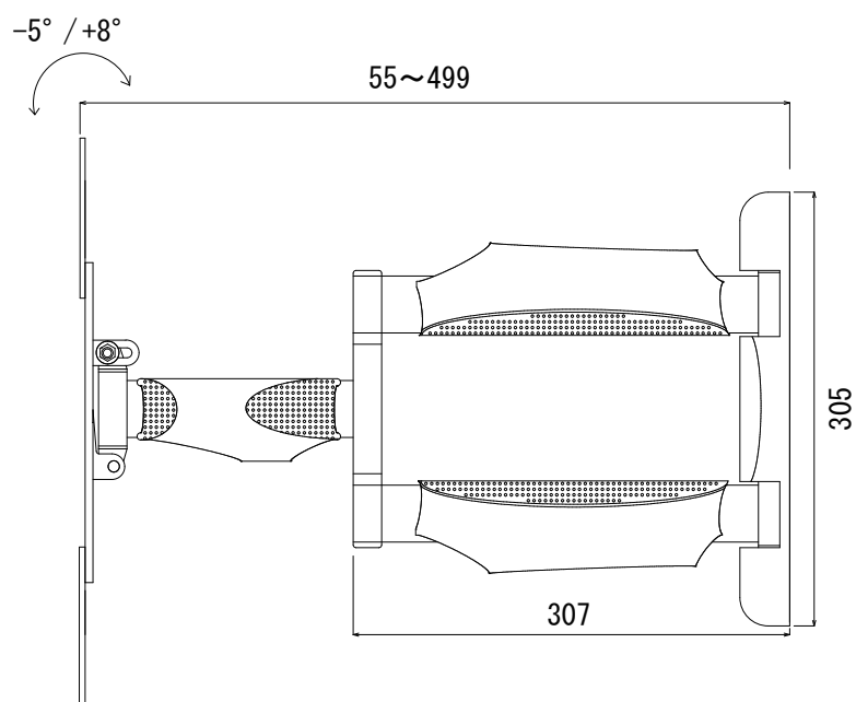
【側面 カバー有/アタッチメント有】
