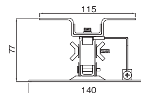
【正面図】
