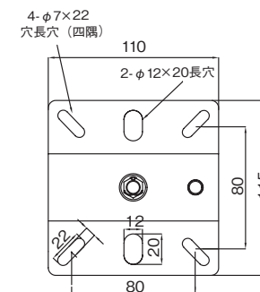
【天井ベース】
