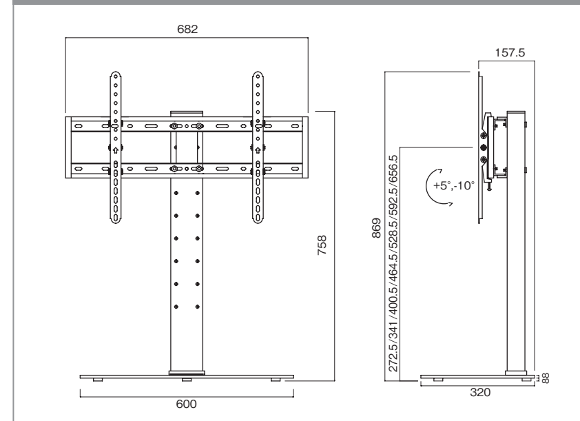
寸法図 (単位 mm)
