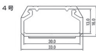
MML型番寸法表
