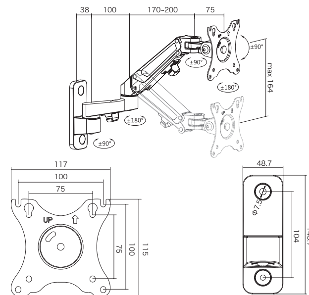
寸法図(単位 mm)
