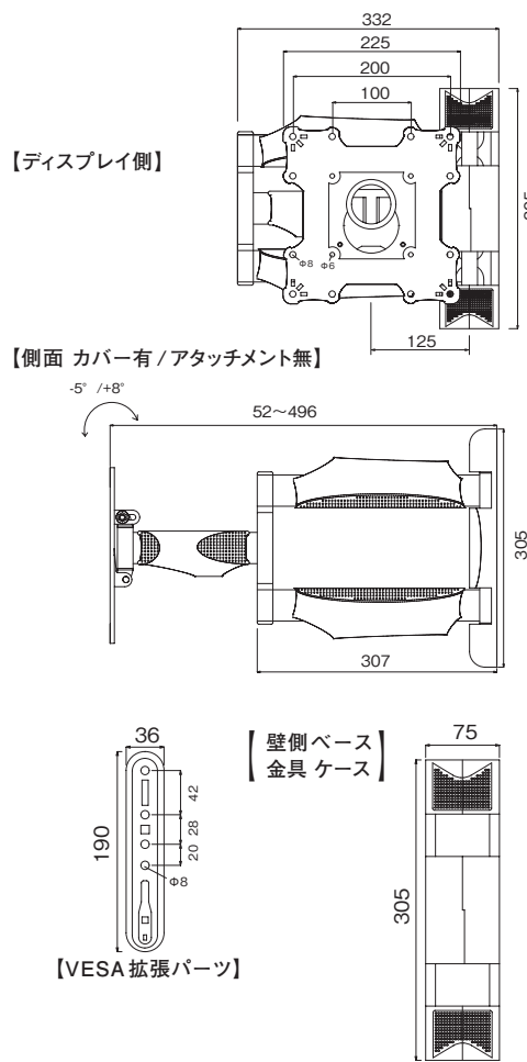
寸法図(単位 mm)
