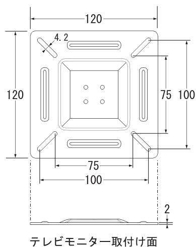
【モニター側】
