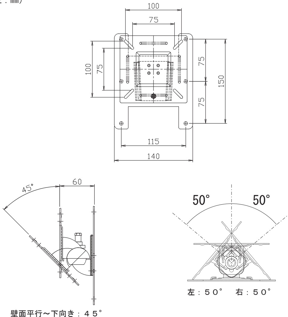
【側面】
